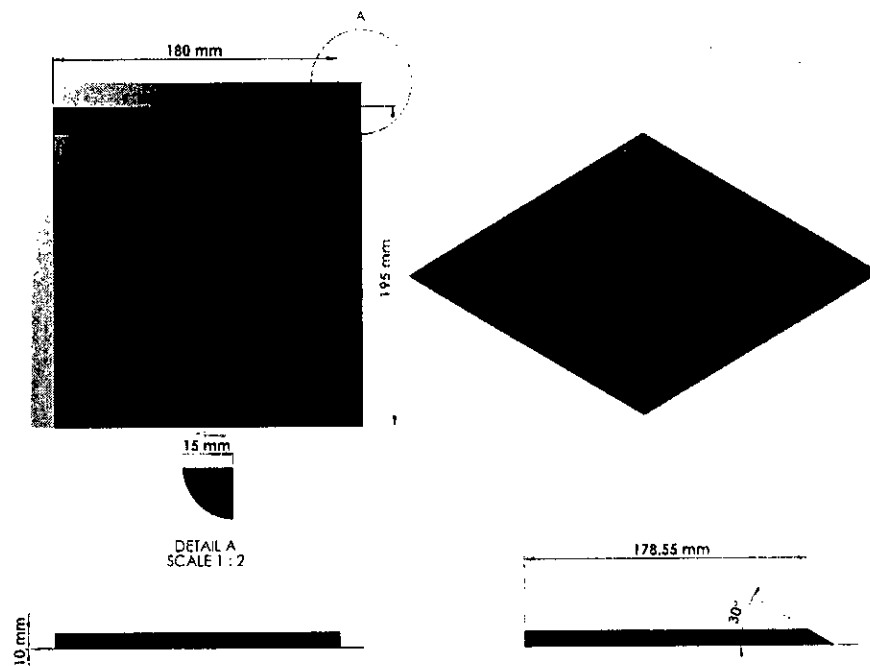
Hình vẽ cấu tạo Kho chứa điều vàng và điều bạc sau khi điều chỉnh
