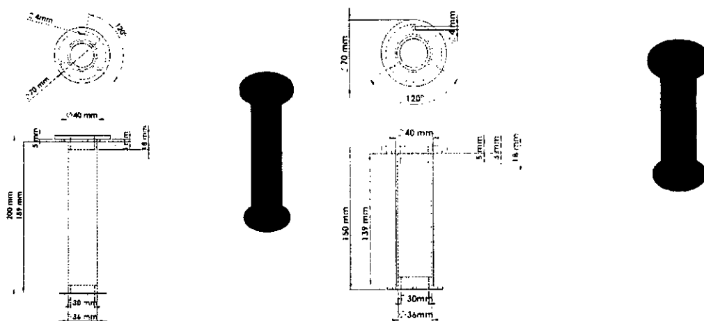
Hình vẽ thiết kế chi tiết của các trụ đặt quả điều sau khi điều chỉnh
